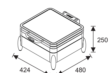
W20-2302T Indukčná ohrevná nádoba W07-2304B Multifunkčná základňa Výška s otvoreným vekom: 687mm
