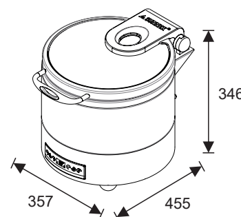
W07-2802T Indukčná ohrevná nádoba W07-2801B Electrická základňa Výška s otvoreným vekom: 730mm
