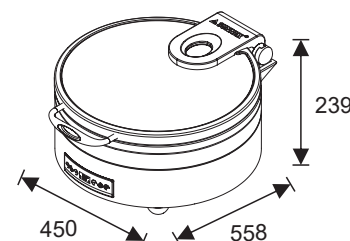
W07-3602T Indukčná ohrevná nádoba W07-3601B Electrická základňa Výška s otvoreným vekom: 715mm
