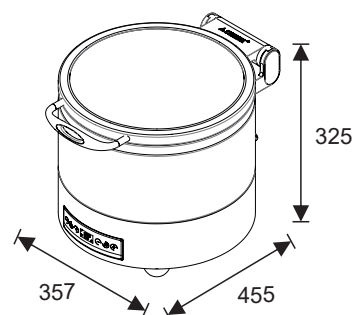
W20-2802T Indukčná ohrevná nádoba W07-2801 Electrická základňa Výška s otvoreným vekom: 730mm
