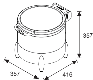
W20-2802T Indukčná ohrevná nádoba W07-2804B Multifunkčná základňa Výška s otvoreným vekom: 762mm
