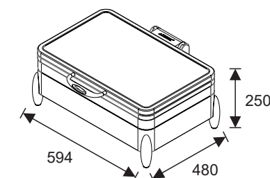
W20-1102T Indukčná ohrevná nádoba W07-1104B Multifunkčná základňa Výška s otvoreným vekom: 687mm
