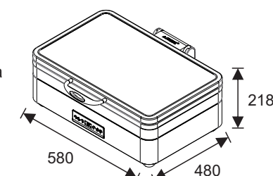
W20-1102T Indukčná ohrevná nádoba W07-1101B Elektrická základňa Výška s otvoreným vekom: 655mm
