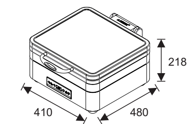
W20-2302T Indukčná ohrevná nádoba W07-2301B Elektrická základňa Výška s otvoreným vekom: 655m
