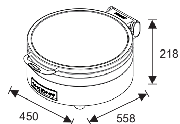
W20-3602T Indukčná ohrevná nádoba W07-3601B Electrická základňa Výška s otvoreným vekom: 715mm
